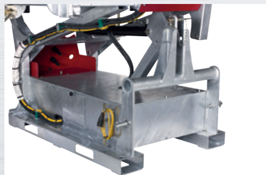
Dreipunkt Cat II, Stapleraufnahme, Hubwagenaufnahme, Anschraubpunkte für Bodenbefestigung
