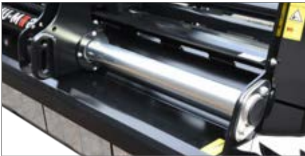
Le déport latéral hydraulique est assuré par des tubes de manœuvre à coussinets plastique pour un fonctionnement à faible usure en utilisation permanente.
