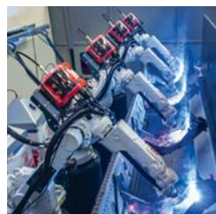
12 îlots de soudage robotisés.
